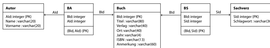
Abbildung 1: Datenbankschema für Literatur
